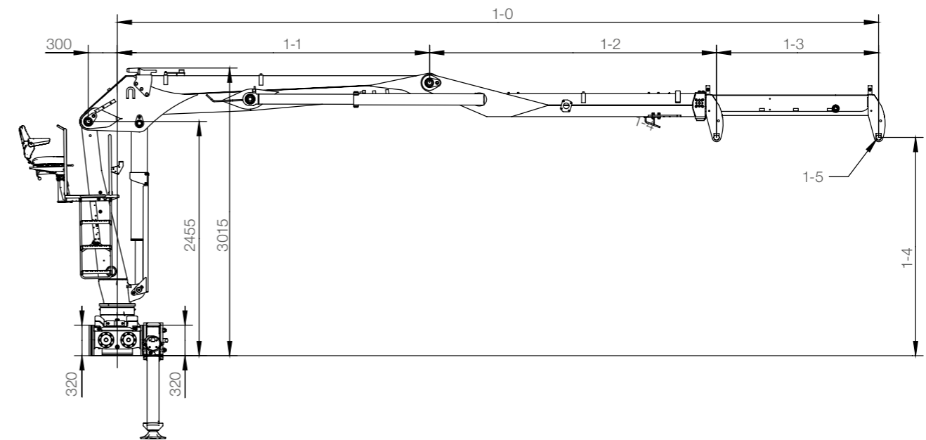
Vista laterale
