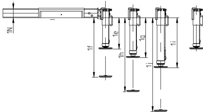
Hydraulisk støtteben
