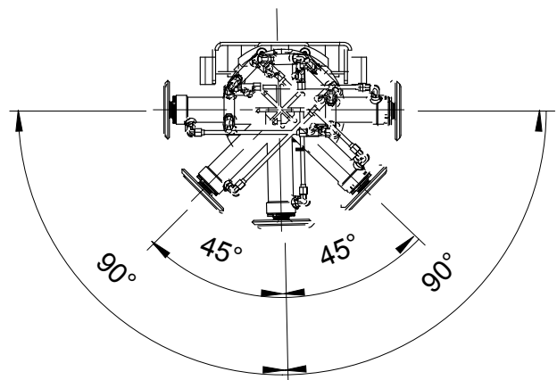
Parkeringsposition for opsvingbar støtteben
